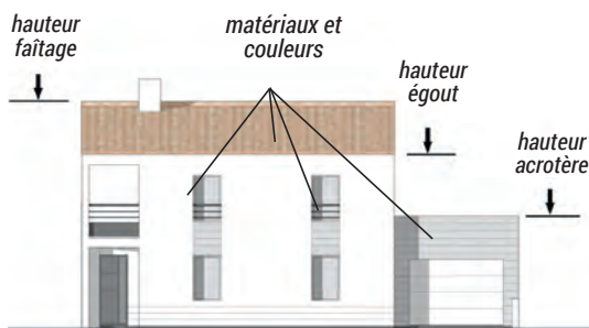
La façade EST
