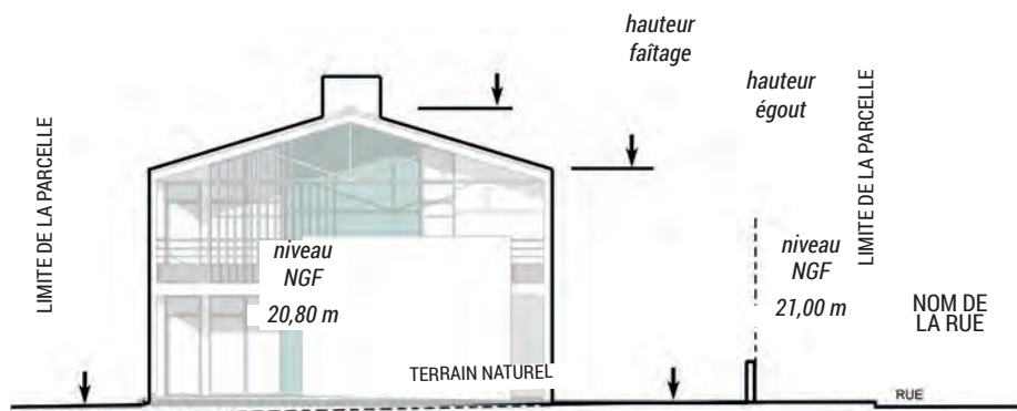
PCMI3 - Le plan de coupe
